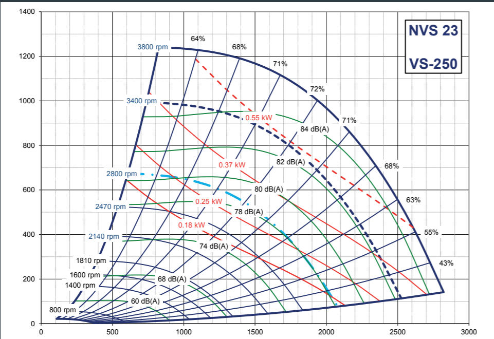
Fan performance NVS 23
