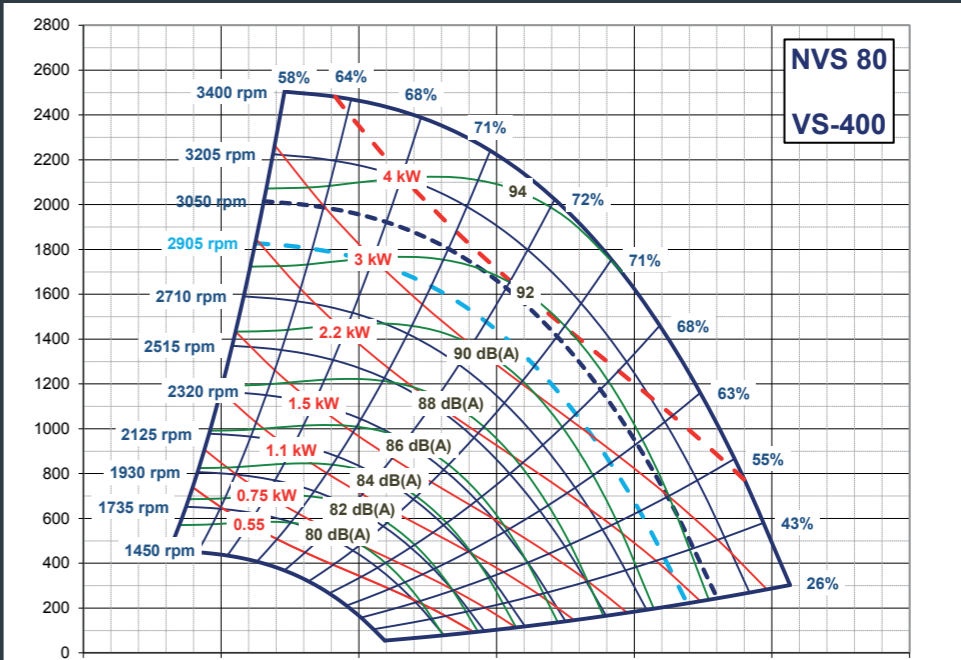
Fan performance NVS 80
