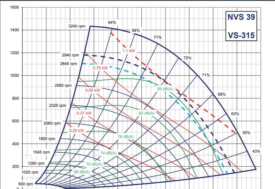
Fan performance NVS 39
