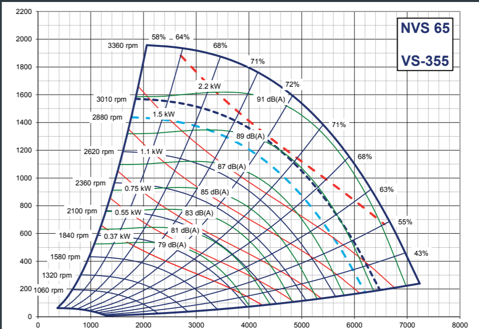
Fan performance NVS 65
